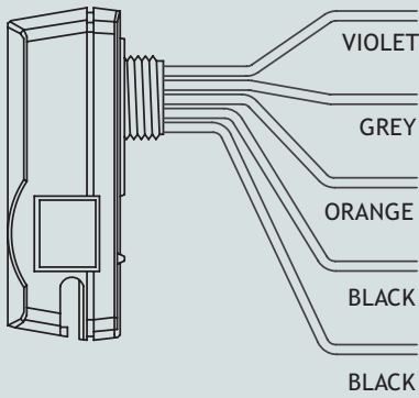
ENCELIUM I/O MODULE
